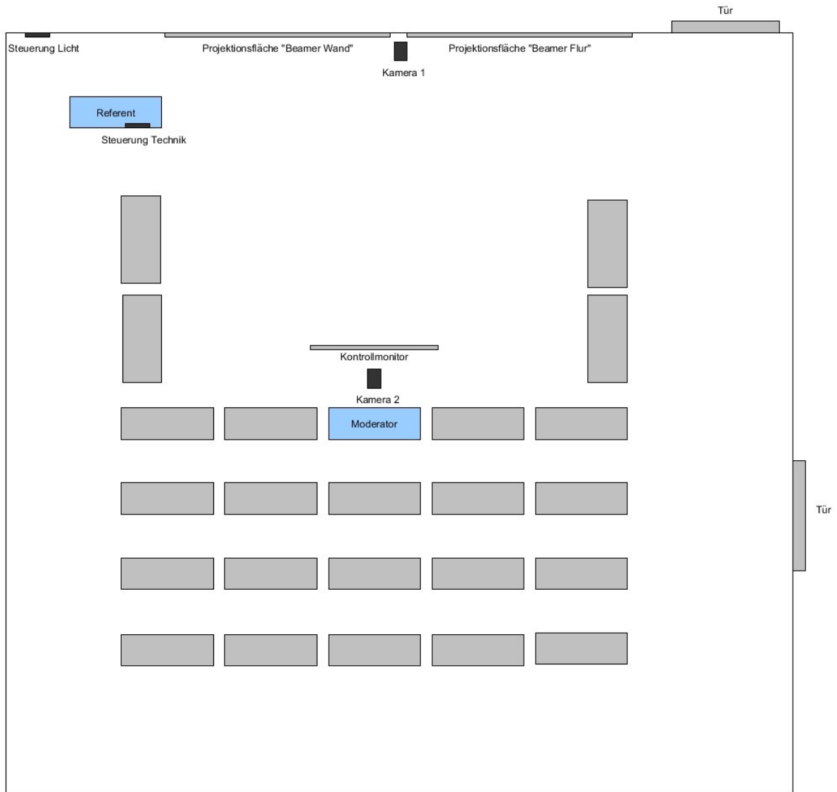
Abbildung 1: Übersicht Videokonferenzraum
